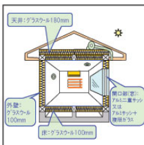
省エネ基準を満たす住宅のイメージ (戸建木造住宅・東京の例)
